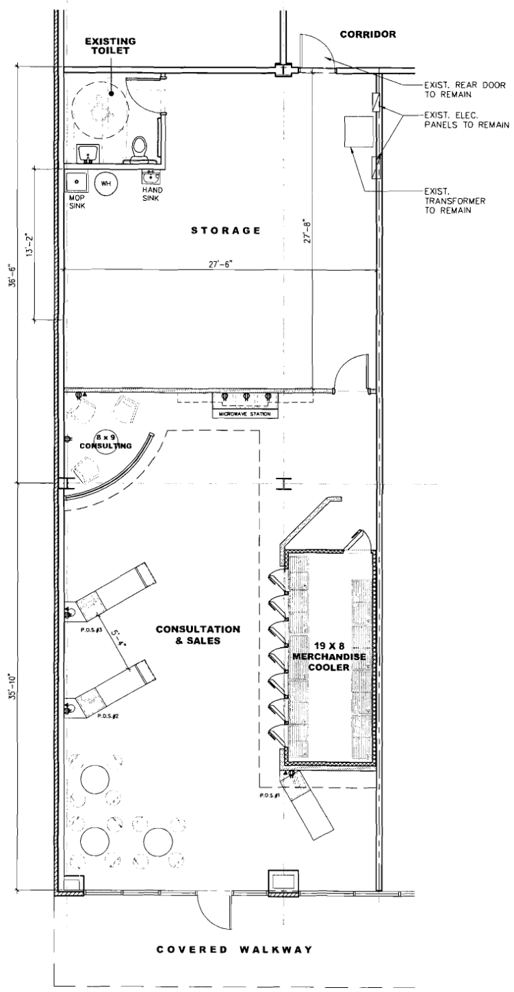
E SCHEMATIC PLAN SCALE: 1/4" = 1'-0"
